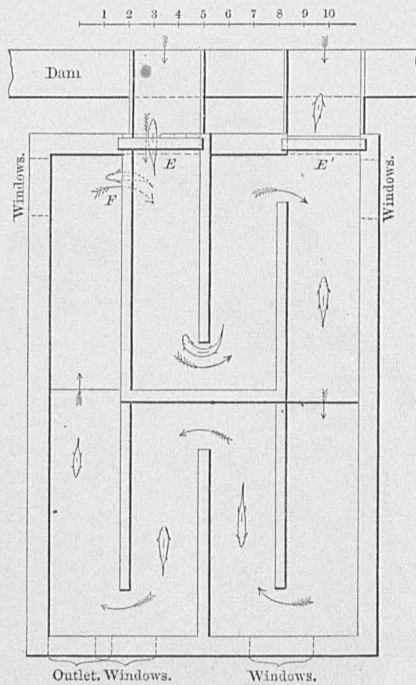
Fig. 1. Plan.
