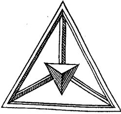
Inscriptum tetraëdron tetraëdro.
