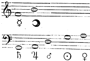
Ecce: Comparatio Ptolemaei.
