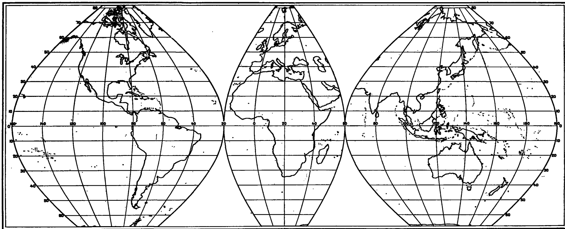
FIG. 80 - SINUSOIDAL OR MERCATOR EQUAL-AREA PROJECTION
