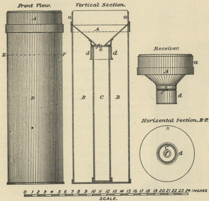
FIG. 11.—Rain gage.
